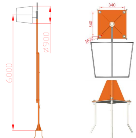
Mástil FAA de 6 metros
